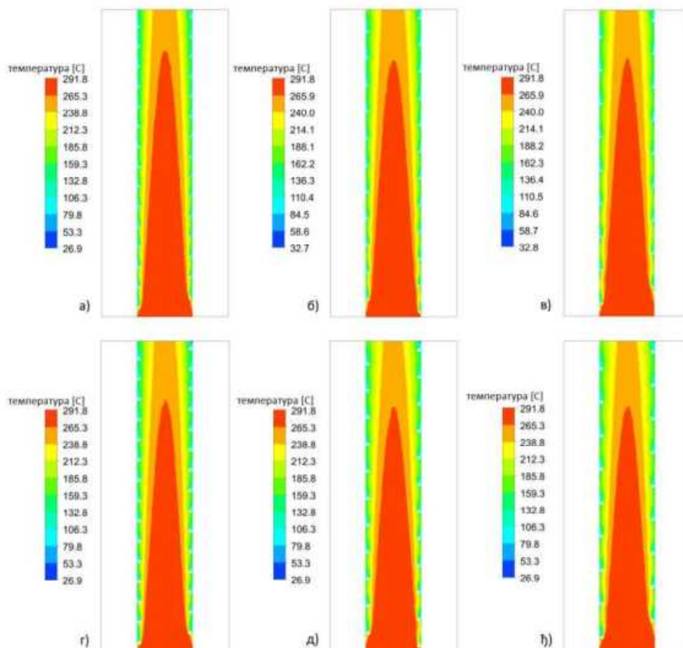
Слика 5.11 | Резултати температурског поља CFD симулација унутар димоводне цеви називног пречника DN80 са турбулаторима у облику жице; а) e=3.5\text{ mm} , r=30\text{ mm} , б) e=3.5\text{ mm} , r=40\text{ mm} , в) e=3.5\text{ mm} , r=50\text{ mm} , г) e=5\text{ mm} , r=30\text{ mm} , д) e=5\text{ mm} , r=40\text{ mm} , б) e=5\text{ mm} , r=50\text{ mm} .
