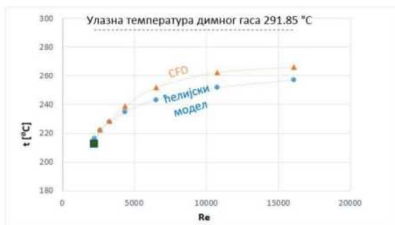
Слика 5.7 | Поређење излазних температура димног гаса предвиђене ћелијским и CFD моделом за празну цев испитних димензија као испитивана цев (Слика преузета из реф. [126]).
