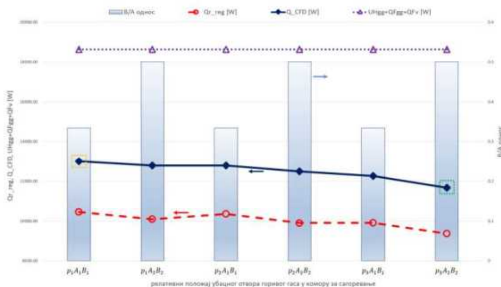
Слика 4.23 | Резултати CFD симулација.
