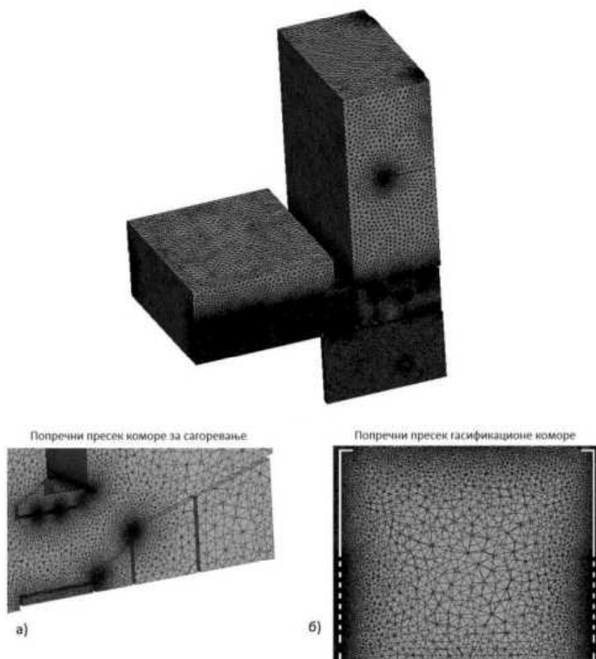
Слика 3.7 | Изометријски приказ изабране фиње мреже са зонама од интереса. а) попречни пресек коморе за сагоревање (поглед са стране), б) попречни пресек гасификационе коморе (поглед одозго).
