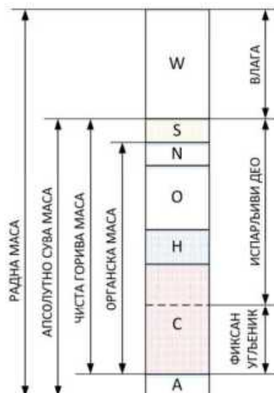
Слика 2.3 | Графички приказ анализе елементарног састава дрвне биомасе.
