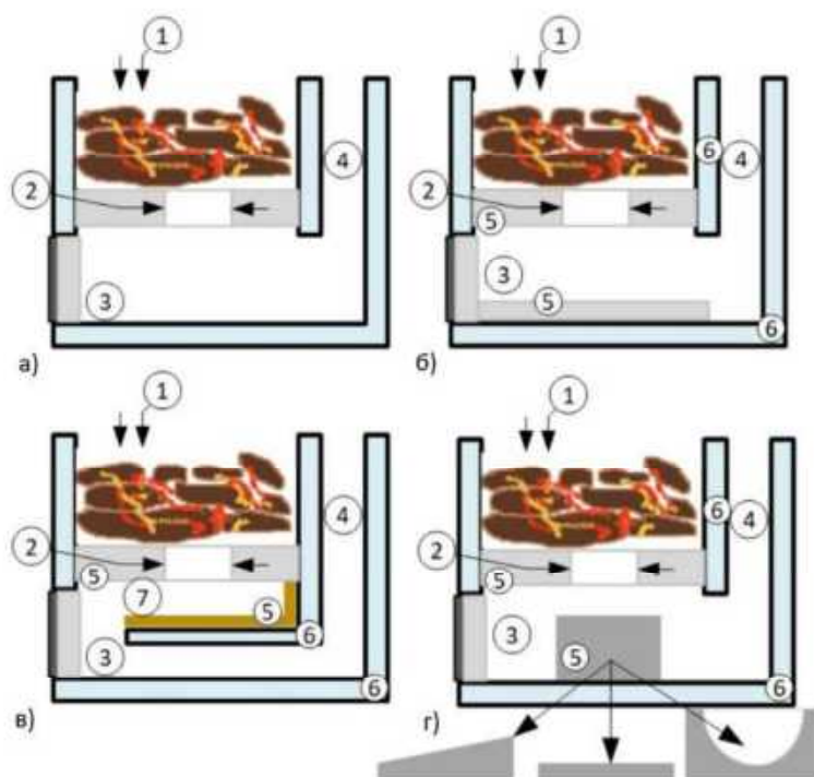
Слика 3.2 | Анализирани конструкције гасификационих котлова са истосмерном гасификацијом огревног дрвета. 1 - примарни ваздух (за гасификацију) и комора за гасификацију, 2 - секундарни ваздух (за сагоревање горивог гаса), 3 - комора за сагоревање, 4 - конвективни део котла, 5 - елементи од ватросталне керамике, 6 - канали за струјање воде, 7 - међукомора (Слика преузета из реф. [11]).
