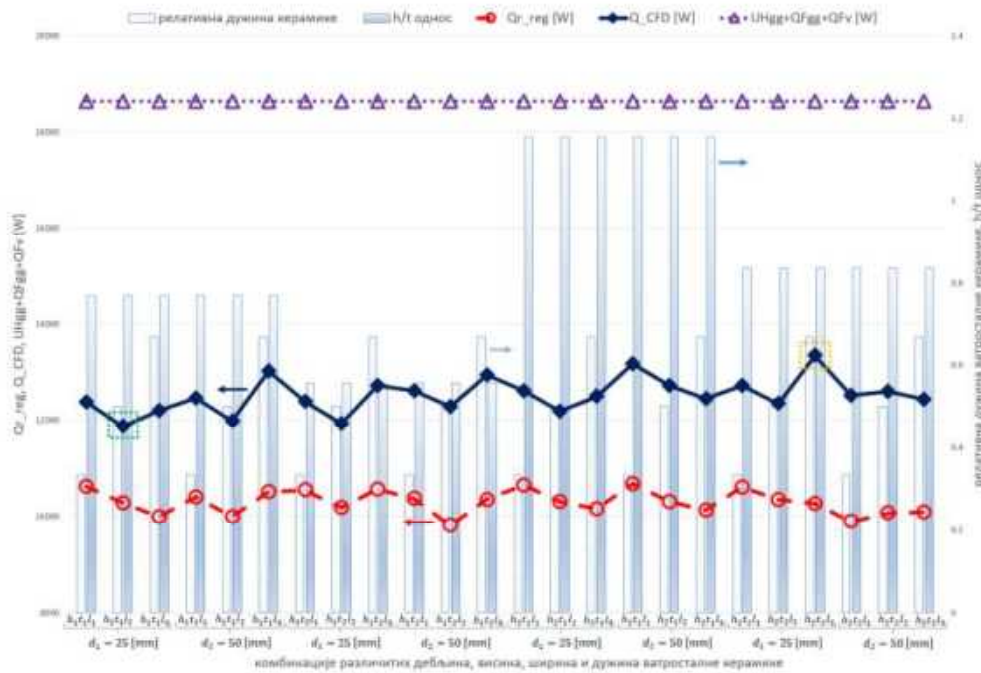
Слика 4.28 | Резултати CFD симулација.
