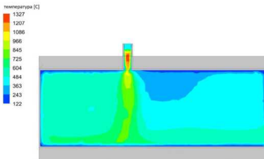
Слика 4.16 | Резултати CFD симулације најповољније варијанте p_5 .
