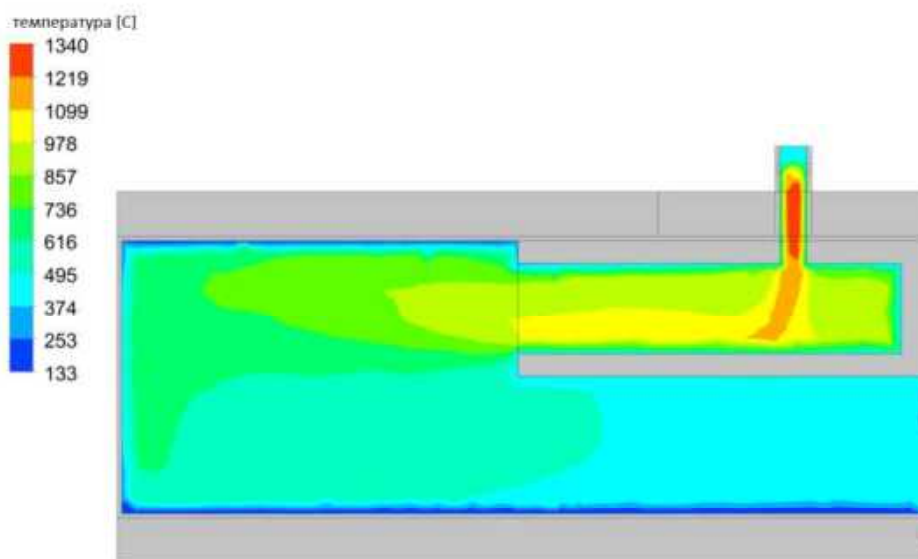
Слика 4.30 | Резултати CFD симулације најнеповољније варијанте d_1h_1t_1l_2 .
