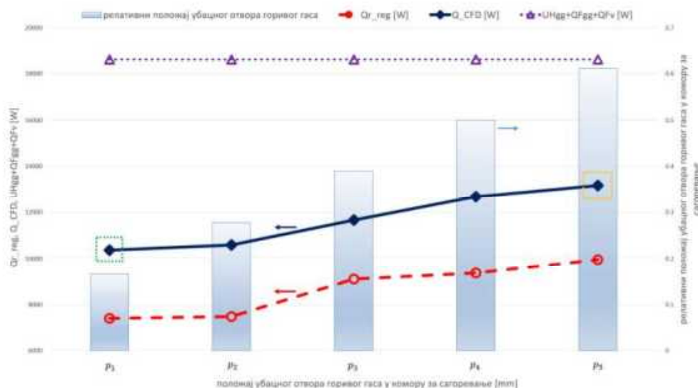
Слика 4.15 | Резултати CFD симулација.
