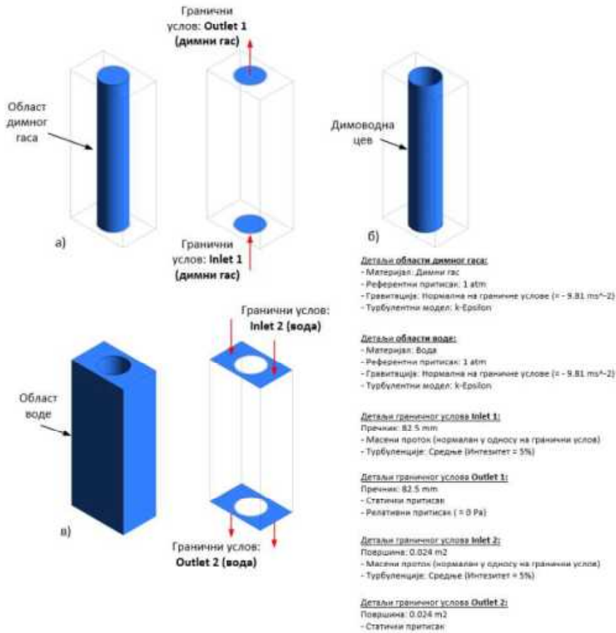
1 Слика 5.5 | Изометријски приказ CFD модела укључујући и детаље о моделу и граничним условима; а) област димног гаса, б) димоводна цев, в – област воде.
