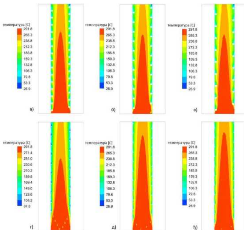
Слика 5.12 | Резултати температурског поља CFD симулација унутар димоводне цеви називног пречника DN80 са турбулаторима у облику жице; а) \epsilon=8\text{ mm} , p=30\text{ mm} , б) \epsilon=8\text{ mm} , p=40\text{ mm} , в) \epsilon=8\text{ mm} , p=50\text{ mm} , г) \epsilon=3.5\text{ mm} , p=40\text{ mm} , \theta=60^\circ , д) \epsilon=3.5\text{ mm} , p=40\text{ mm} , \theta=90^\circ , б) \epsilon=3.5\text{ mm} , p=40\text{ mm} , \theta=120^\circ .
