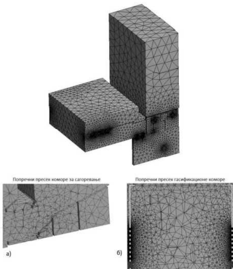
Слика 3.6 | Изометријски приказ првобитно формиране грубе мреже са зонама од интереса. а) попречни пресек коморе за сагоревање (поглед са стране), б) попречни пресек гасификационе коморе (поглед оозго).
