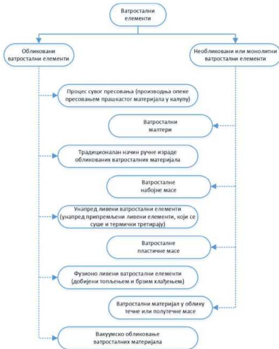
Слика 4.1 | Класификација ватросталних материјала према њиховом облику и начину производње (Слика преузета из реф. [108]).
