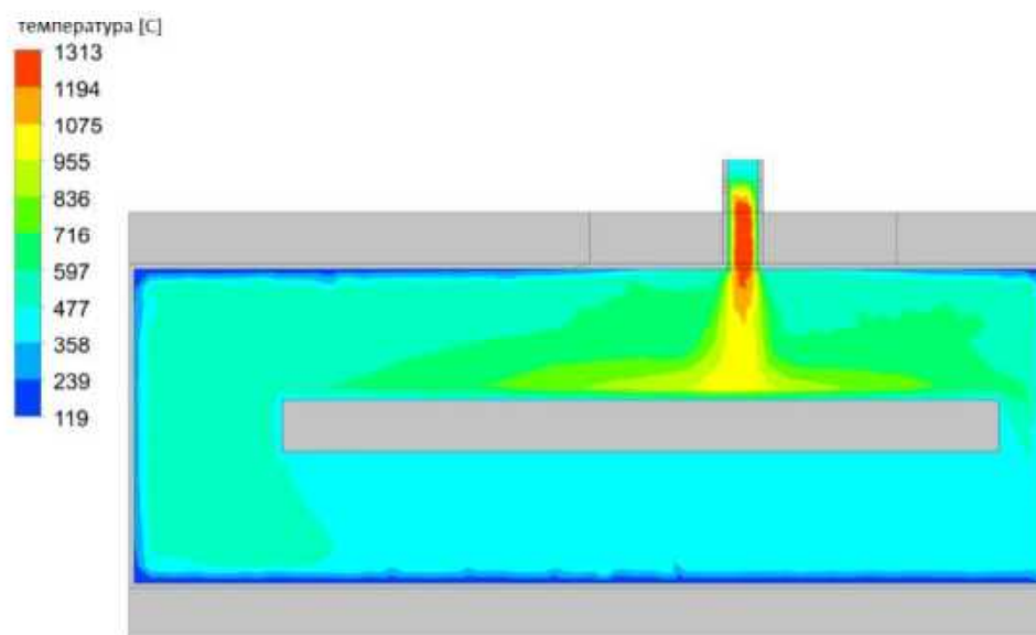
Слика 4.24 | Резултати CFD симулације најповољније варијанте p_1A_1B_1 .
