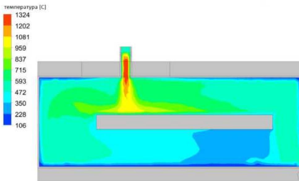
Слика 4.25 | Резултати CFD симулације најнеповољније варијанте p_3A_2B_2 .
