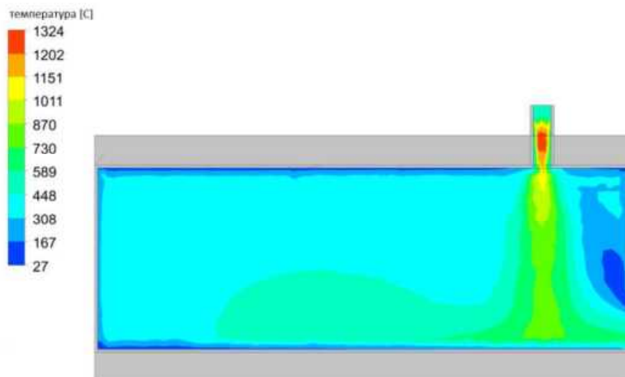
Слика 4.17 | Резултати CFD симулације најнеповољније варијанте p_1 .
