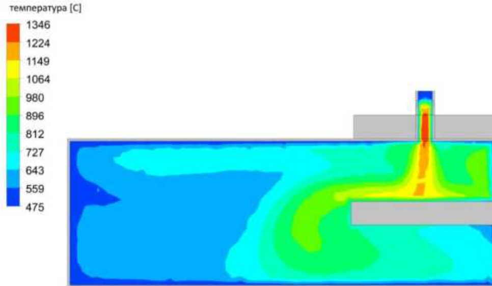
Слика 4.8 | Температурско поље димног гаса.
