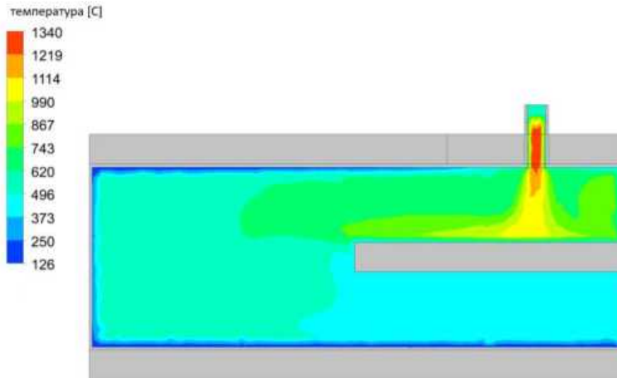
Слика 4.12 | Резултати CFD симулације оптималне варијанте p_1l_3 .
