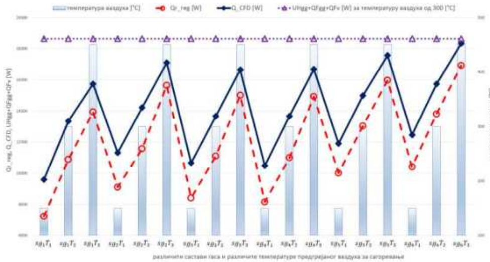
Слика 4.31 | Резултати CFD симулација.
